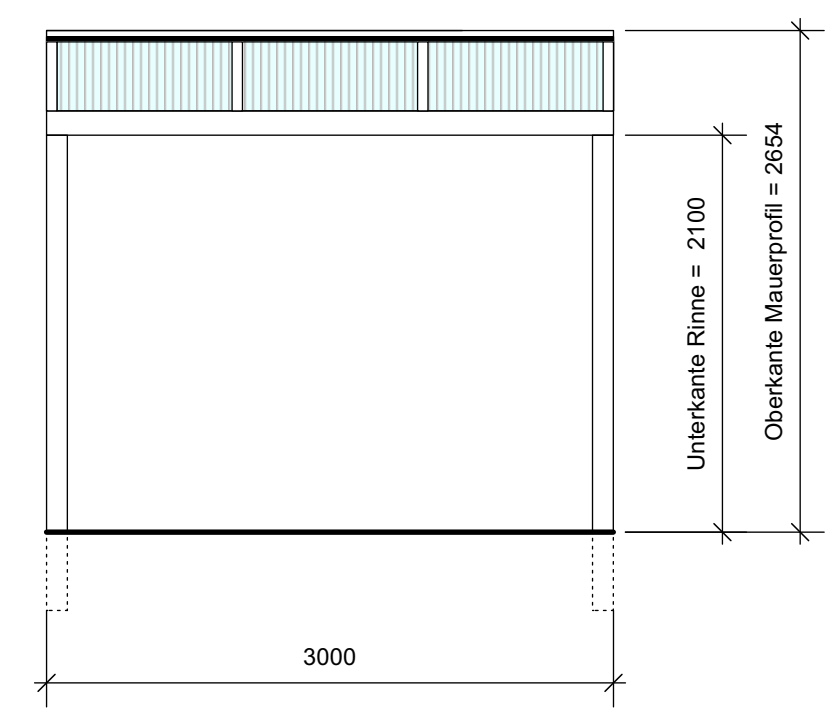
Vorderansicht
