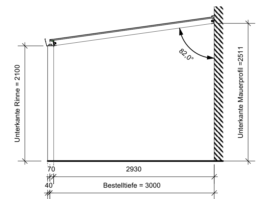
Schnitt
