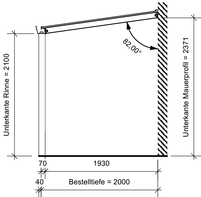
Schnitt
