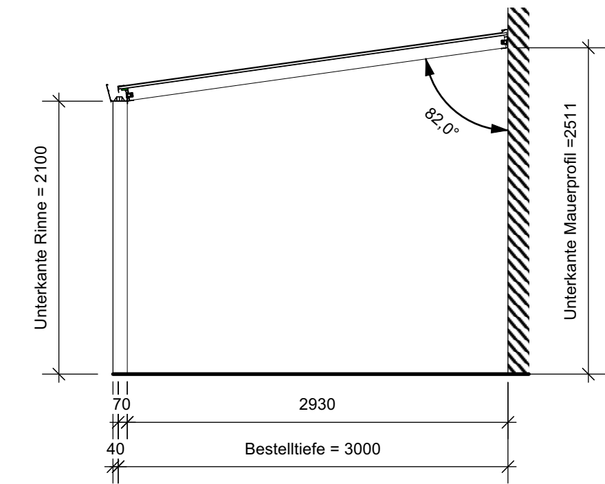
Schnitt
