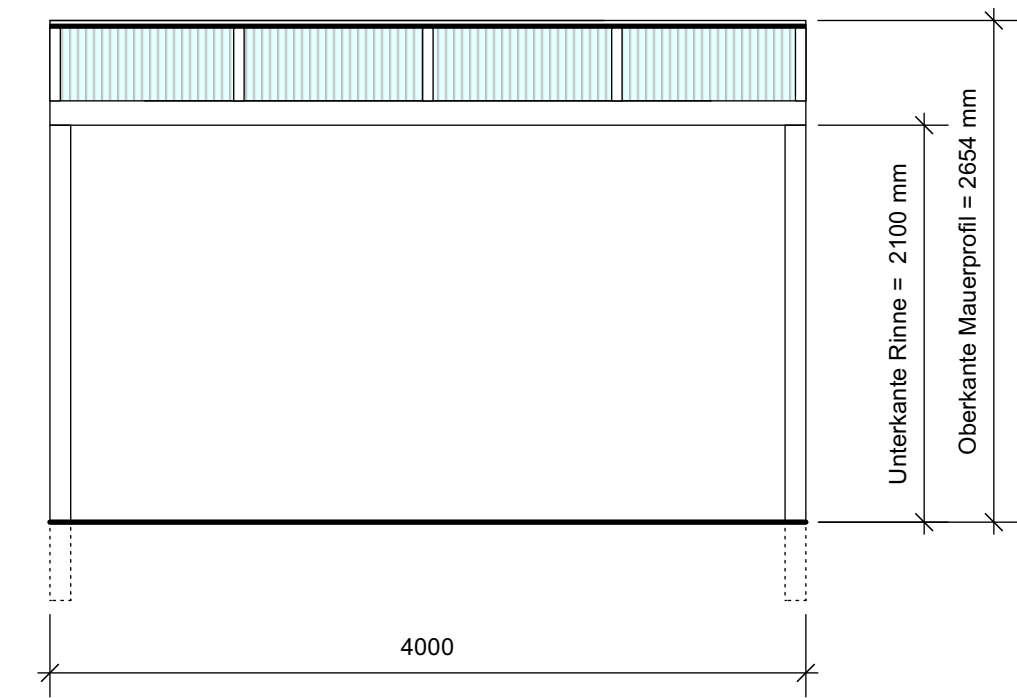
Vorderansicht
