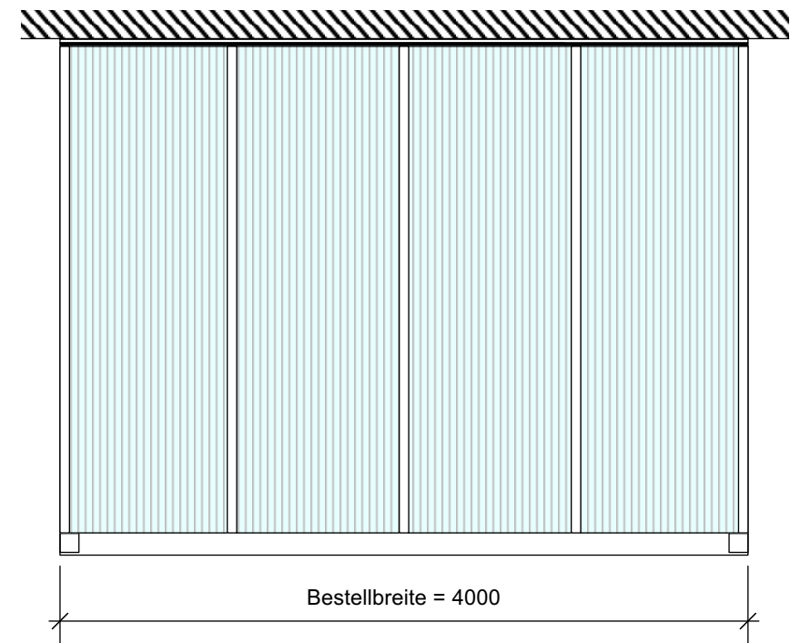
Draufsicht
