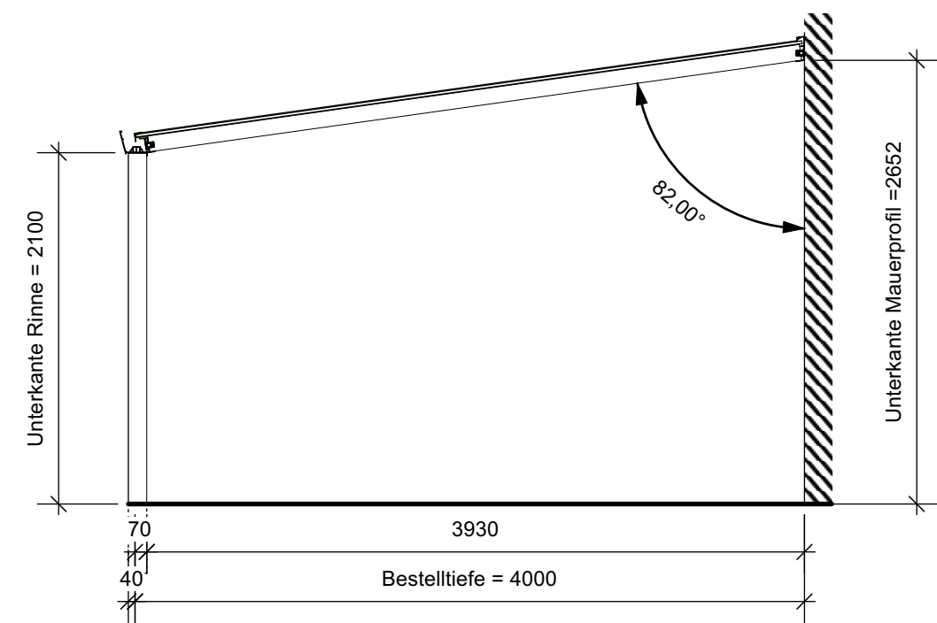
Schnitt
