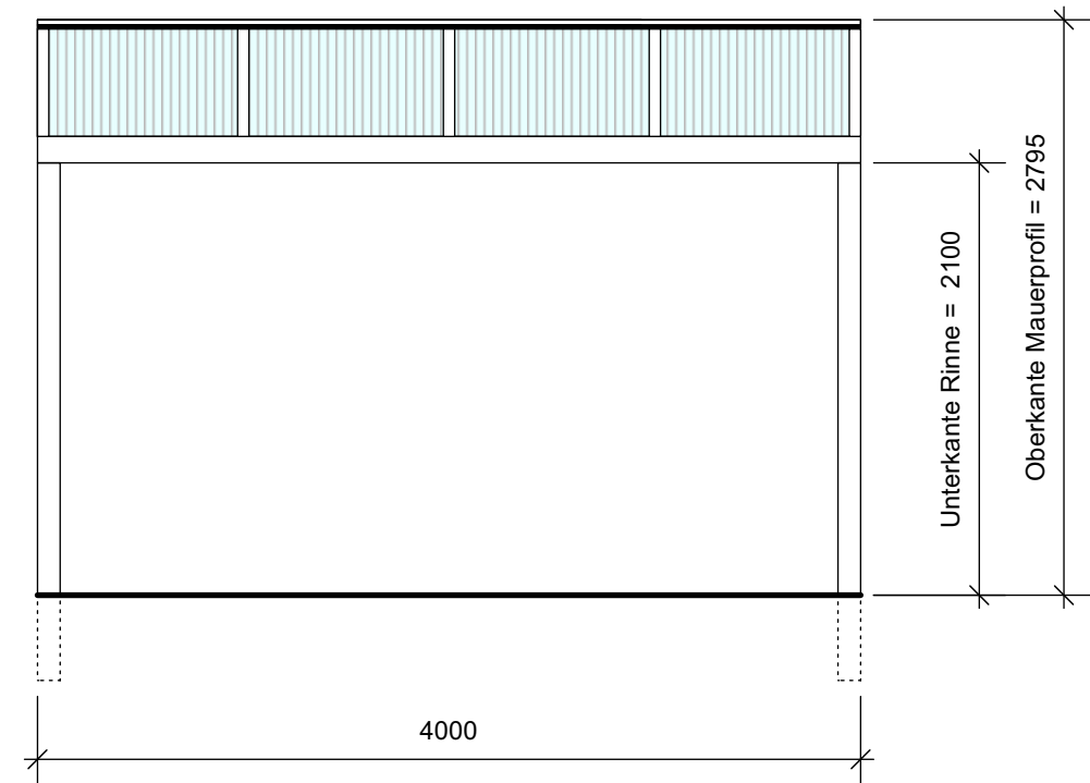
Vorderansicht
