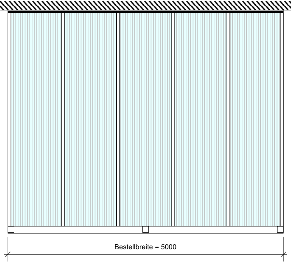
Draufsicht
