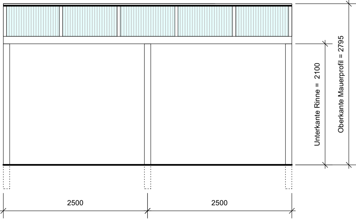
Vorderansicht
