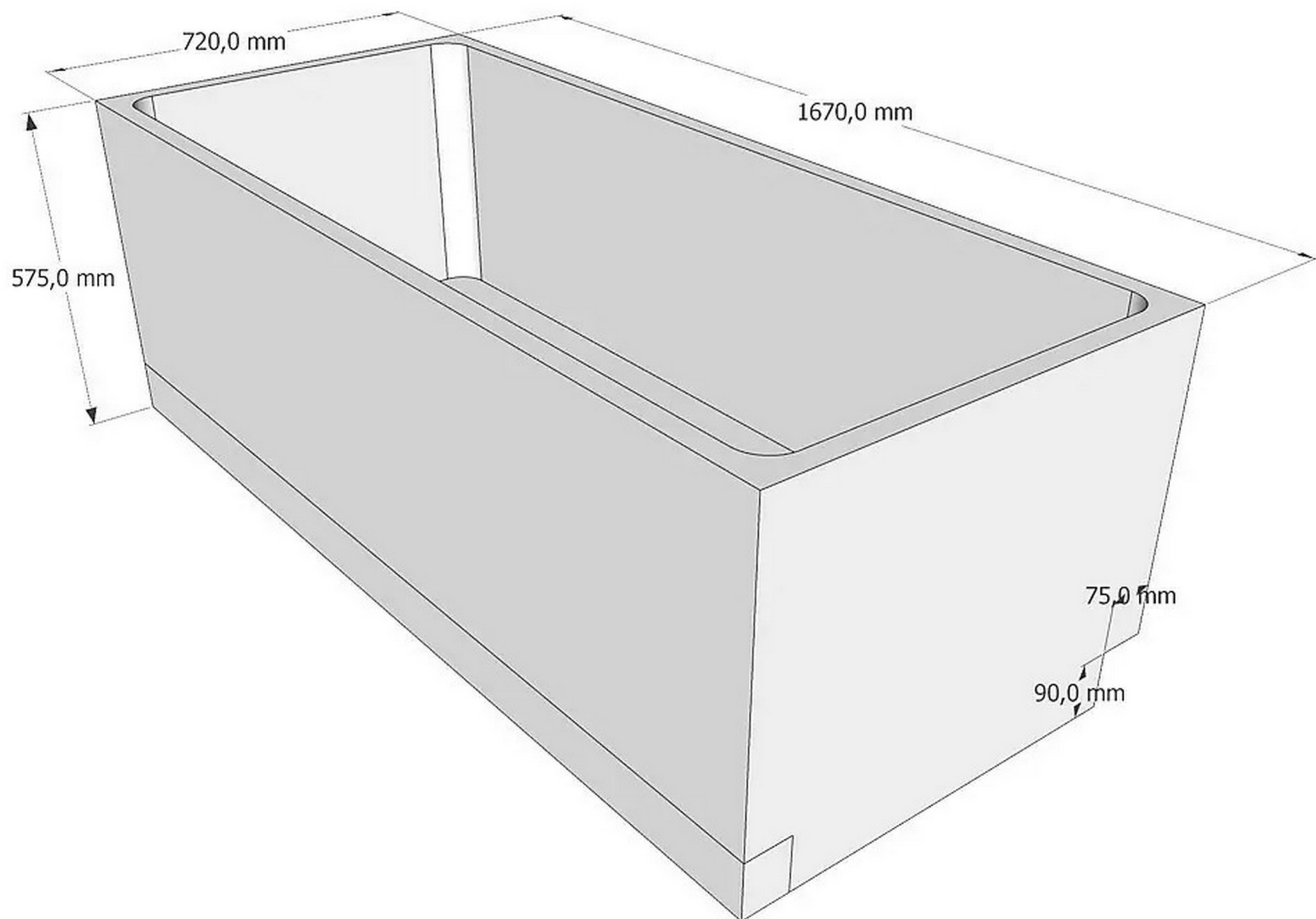
170x75 cm Kaldewei, Bette, Laufen (2xgerade Front) AF Trägerhöhe: 57.5 cm
