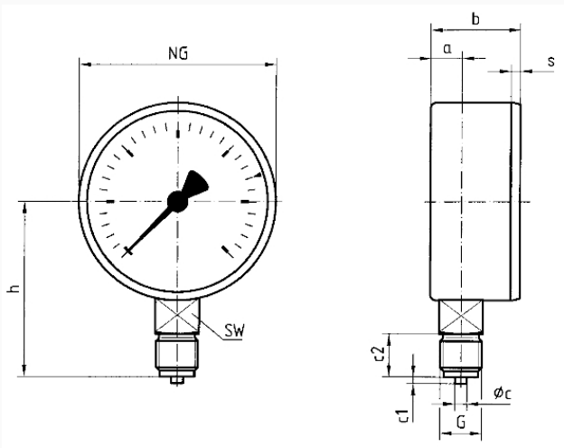
Maße (mm)
