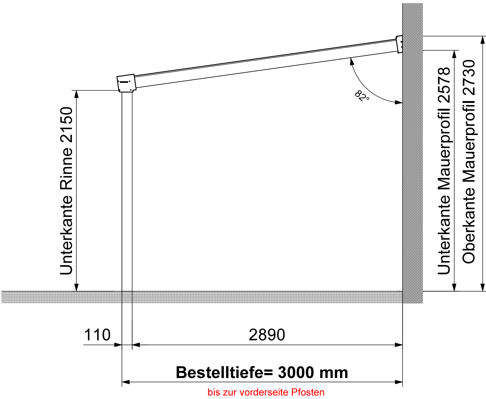
SEITENANSICHT RECHTS
