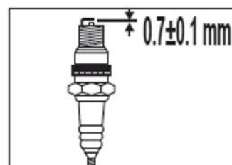
A gyújtógyertya ellenőrzése
