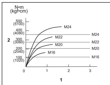
1. Tempo de aperto (segundos) 2. Binário de aperto
