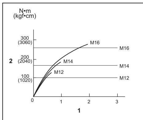
1. Aandraaitijd (seconden) 2. Aandraaimoment
