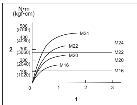
1. Aandraaitijd (seconden) 2. Aandraaimoment
