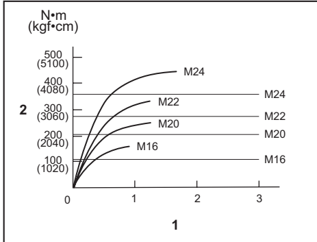
1. Sıkma süresi (saniye) 2. Sıkma torku
