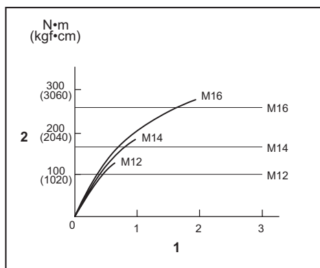
1. Tempo de aperto (segundos) 2. Binário de aperto
