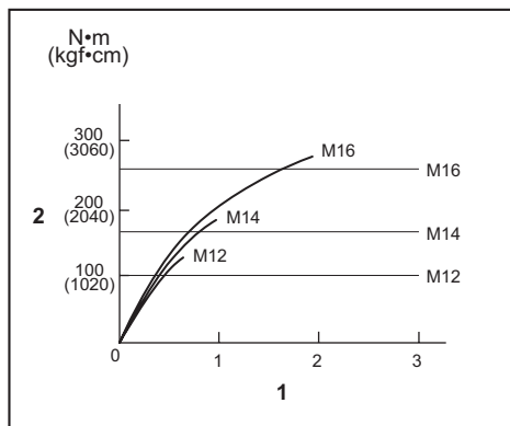
1. Tiempo de apriete (segundo) 2. Par de apriete
