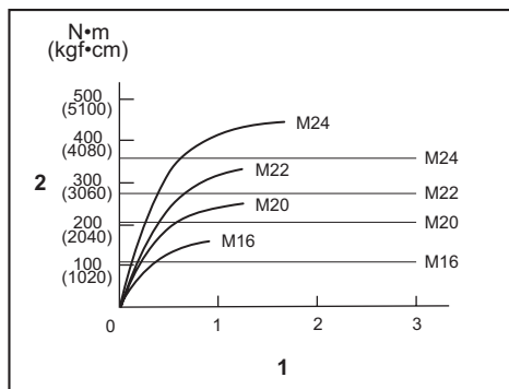
1. Tempo di serraggio (secondi) 2. Coppia di serraggio
