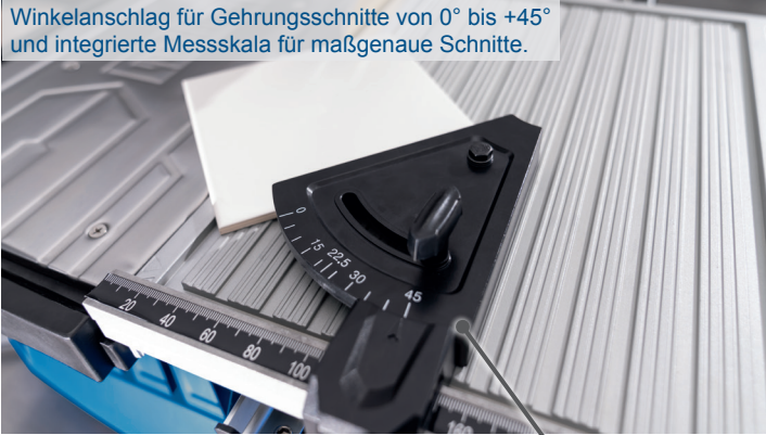
Winkelanschlag
