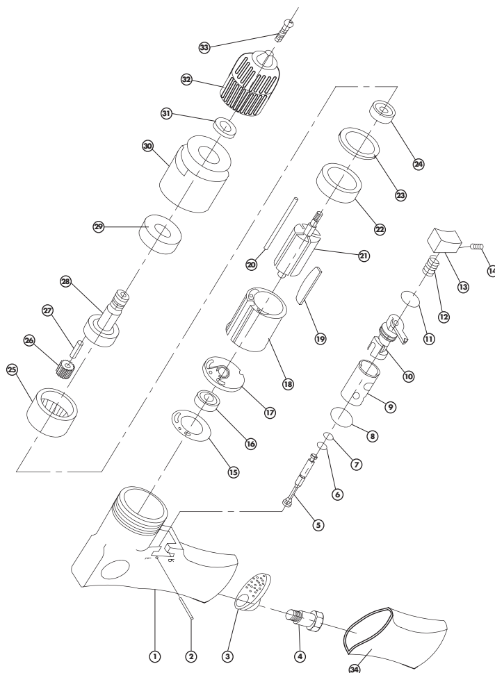
Abb. 3: Explosionszeichnung
