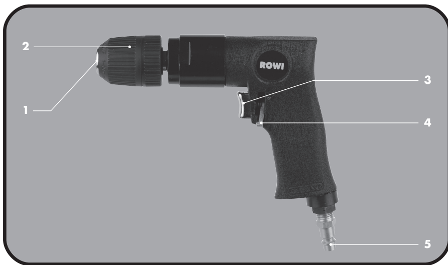
Abb. 1: Geräteübersicht
