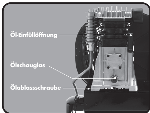
Abb. 3: Öl auffüllen
