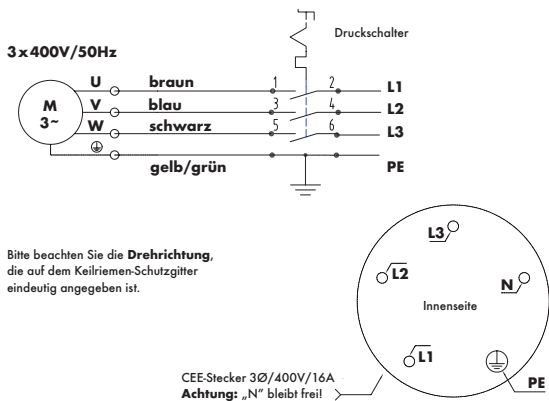
Abb. 9: Schaltplan
