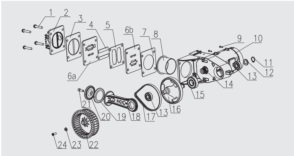
Abb. 5: Explosionszeichnung Motor-Einheit
