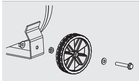
Abb. 1a: Montage Räder
