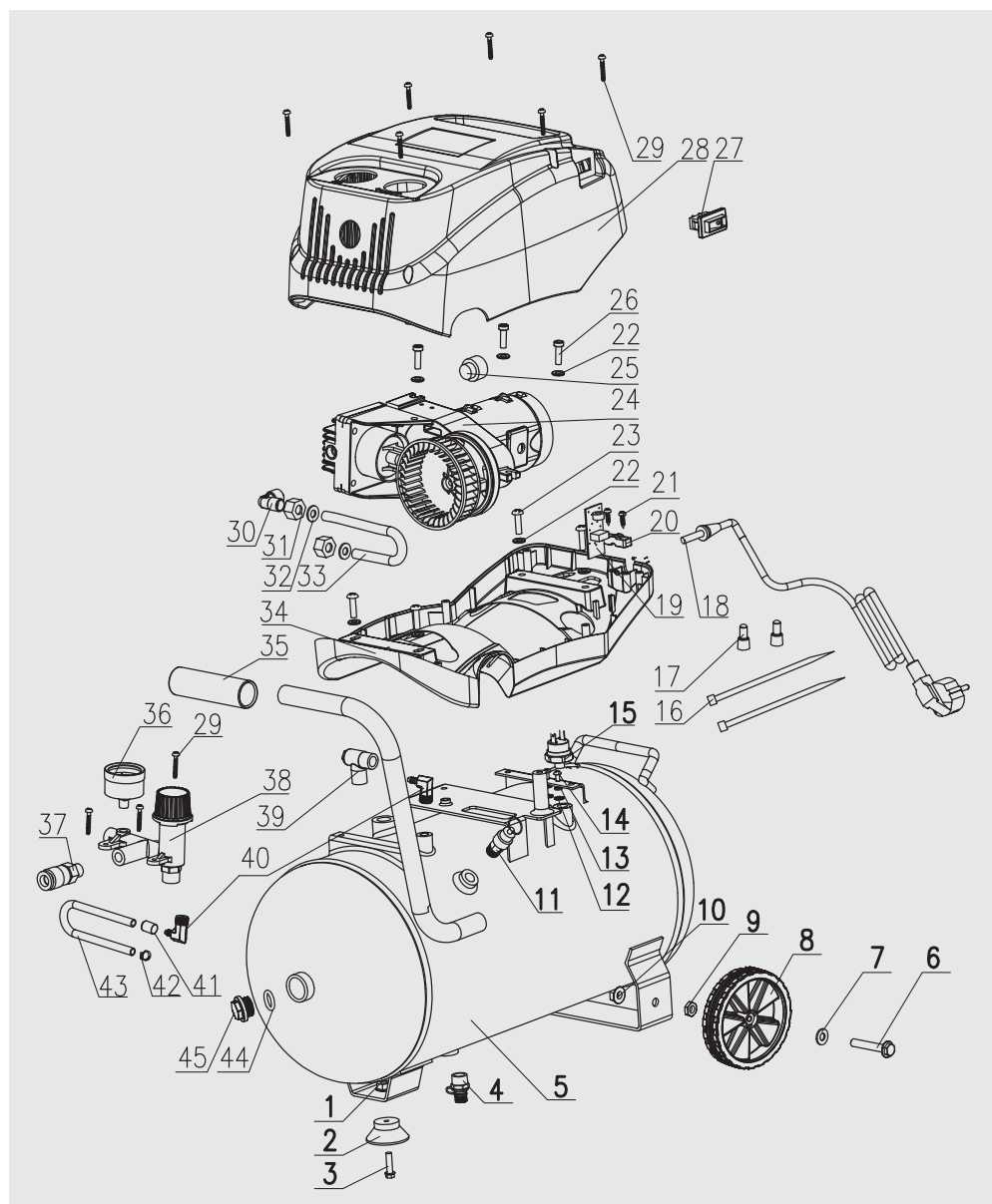
Abb. 4: Explosionszeichnung
