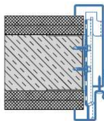
Umfassungszarge Profil 21168
