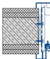
Umfassungszarge Profil 21180
