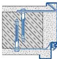
Umfassungszarge Profil 21100
