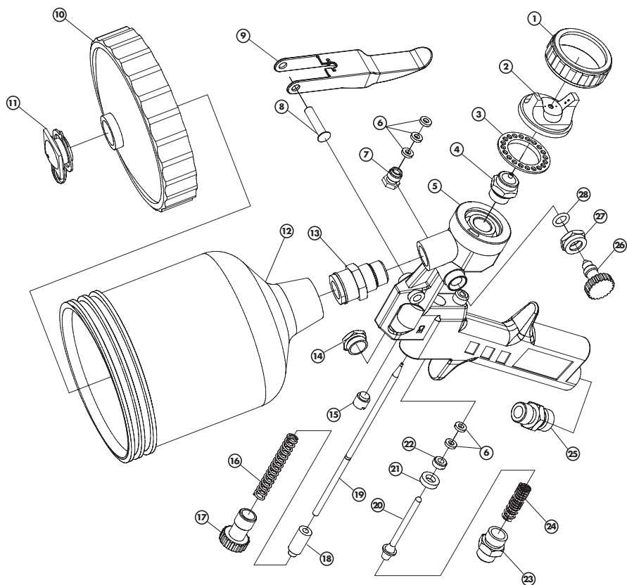
Abb. 3: Explosionszeichnung
