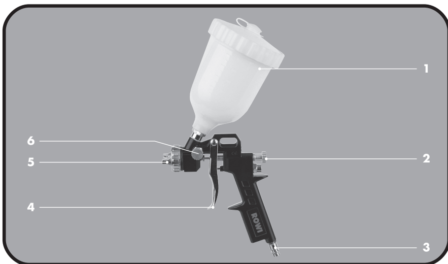
Abb. 1: Geräteübersicht
