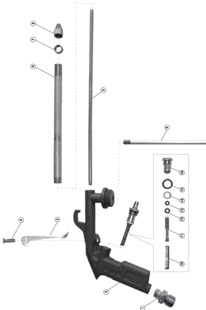
Abb. 3: Explosionszeichnung
