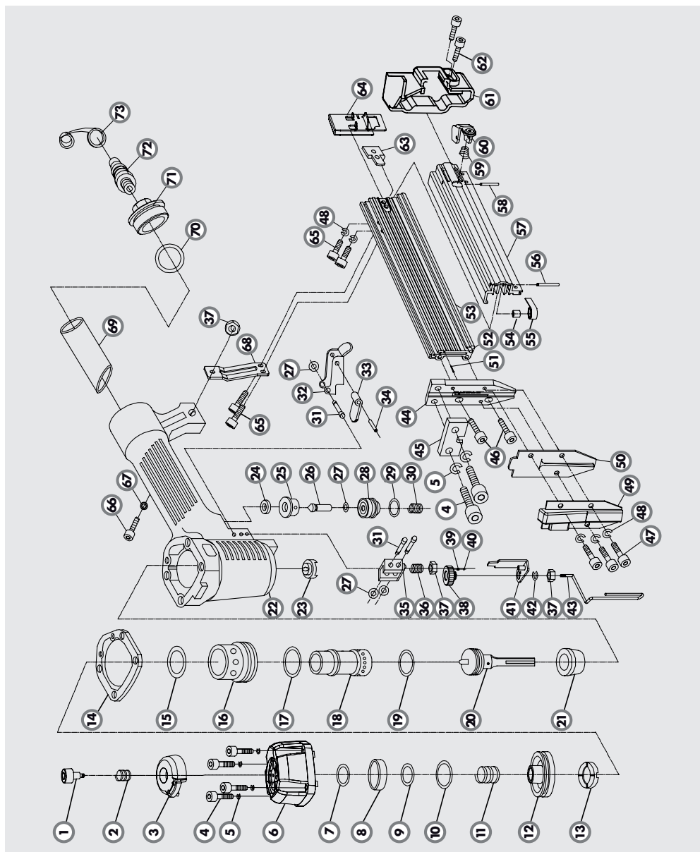
Abb. 2: Explosionszeichnung
