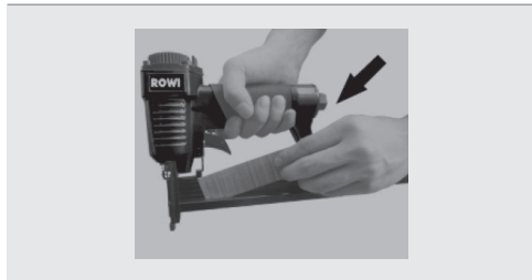
Abb.3: Magazin schließen
