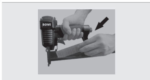
Abb.2: Magazin laden
