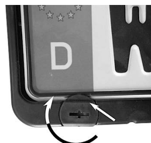
Bild 5: Halterung geschlossen
