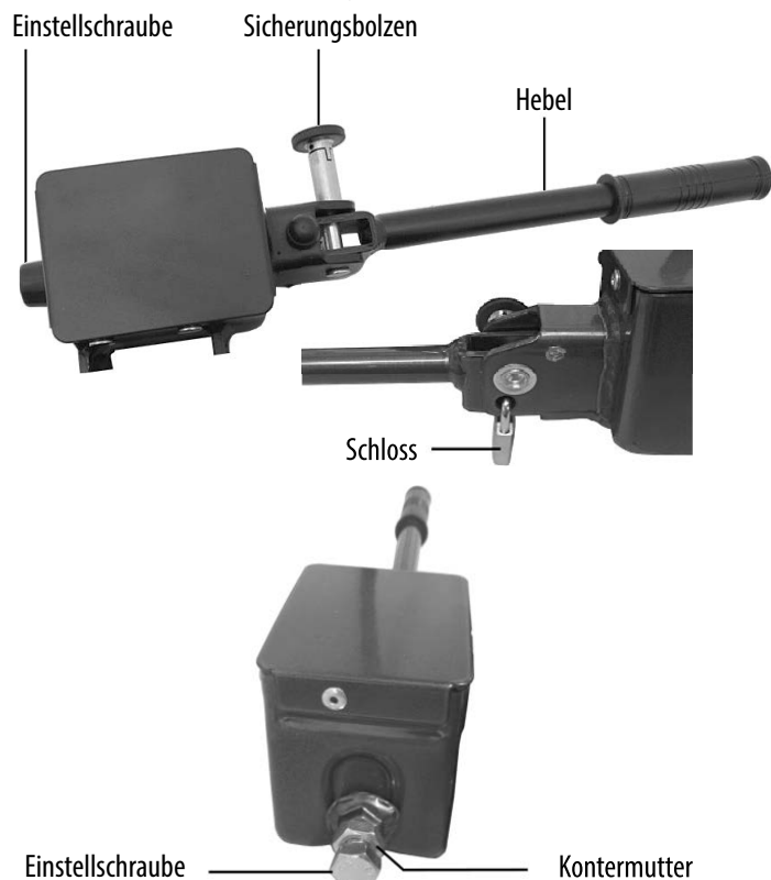
Bild 6: Schnellverschluss
