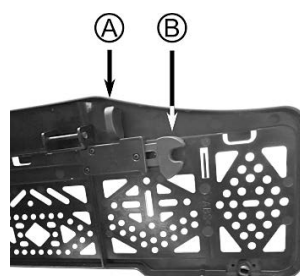
Bild 10: Verriegelung
