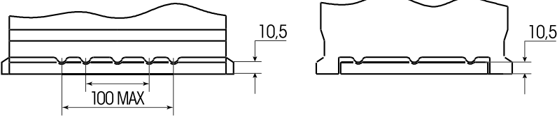
Bodenleiste B13
