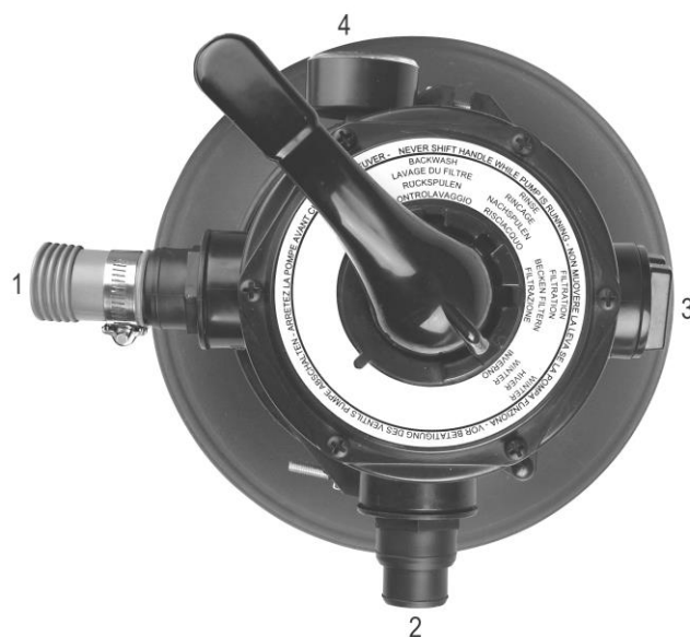
1. Alimentation de la pompe (Pump) 2. Écoulement vers la piscine (Pool) pour le mode filtration 3. Sortie des eaux usées (Waste) pour le rinçage à contre-courant 4. Manomètre
