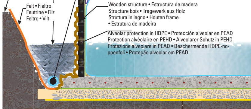
Peripheral drainage • Drenaje periférico Drain périphérique • Periphäre drainage Drenaggio periferico • Perifere afwatering • Drenagem periférica
