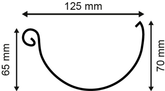
Halbrundrinne 8 tlg Alu Z: 250
