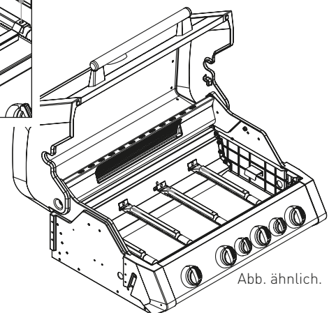
1. Schrauben lösen und Befestigung abheben.
