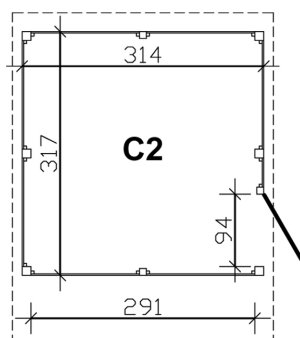
Grundriss Abstellraum C2
