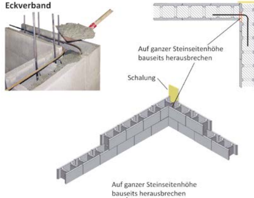
Wandanschluss
