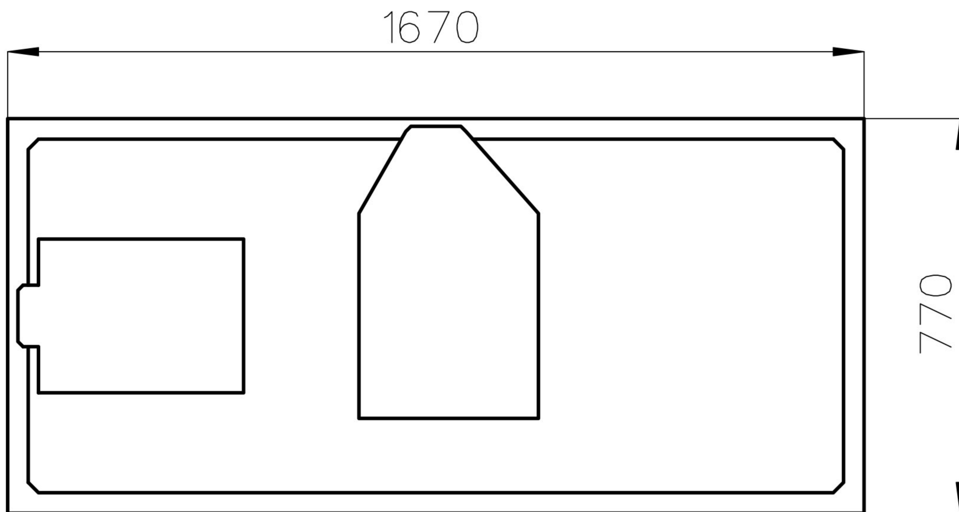
Draufsicht
