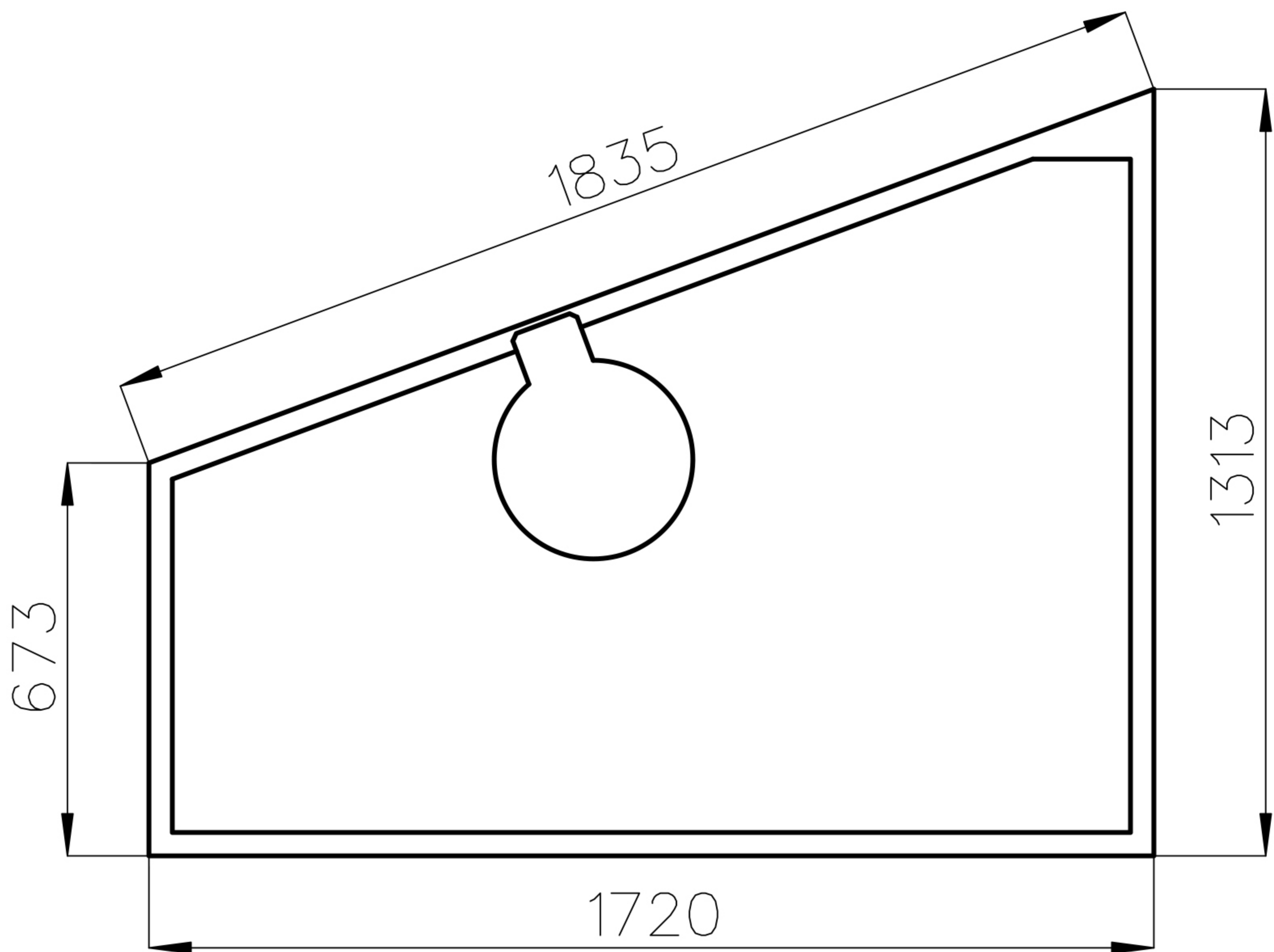
Draufsicht
