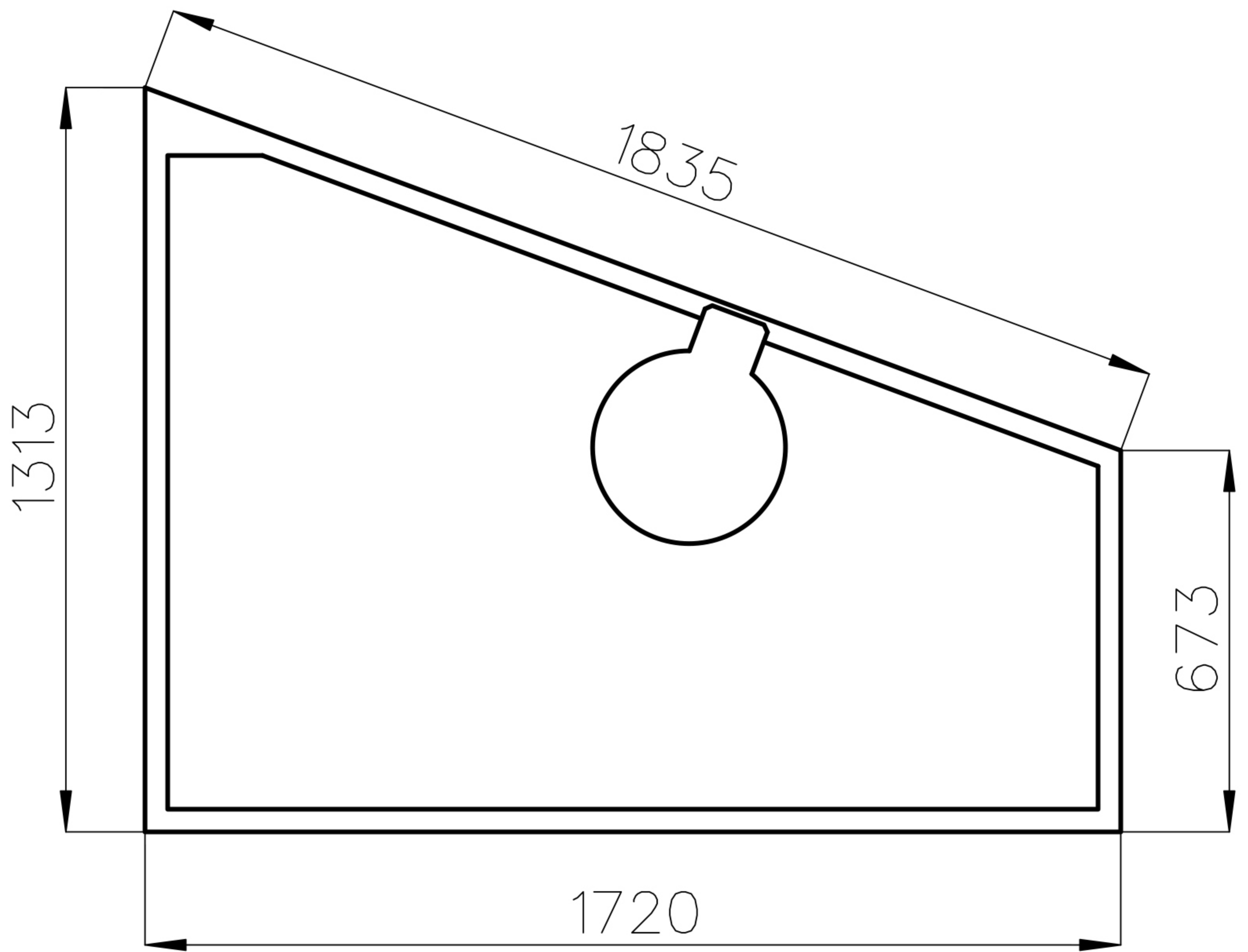
Draufsicht
