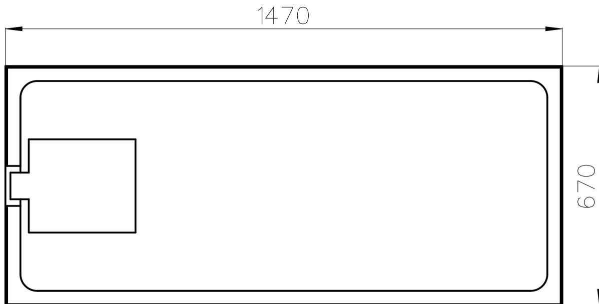
Draufsicht
