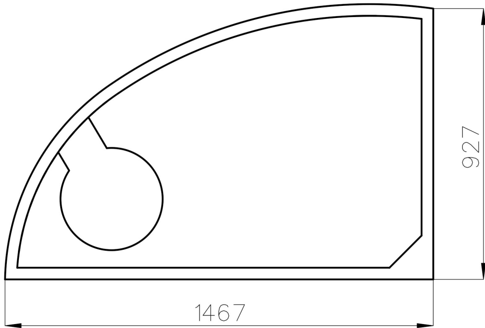
Draufsicht
