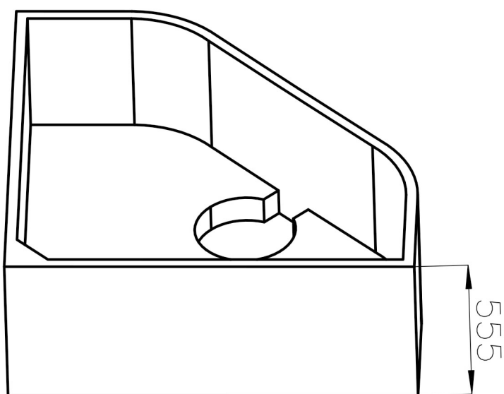
Isometrische Ansicht
