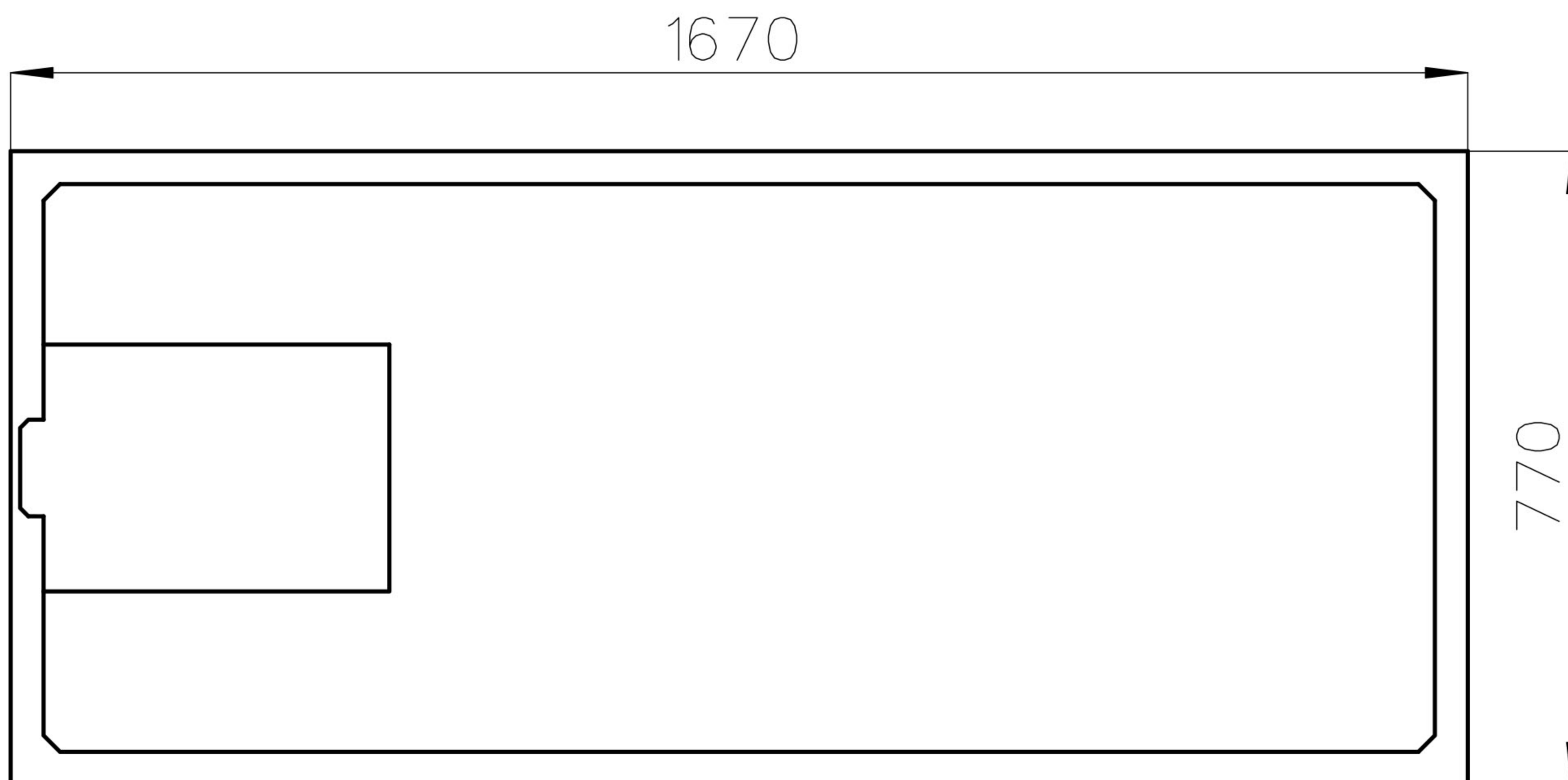
Draufsicht
