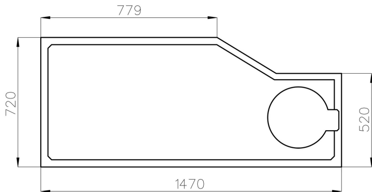
Draufsicht
