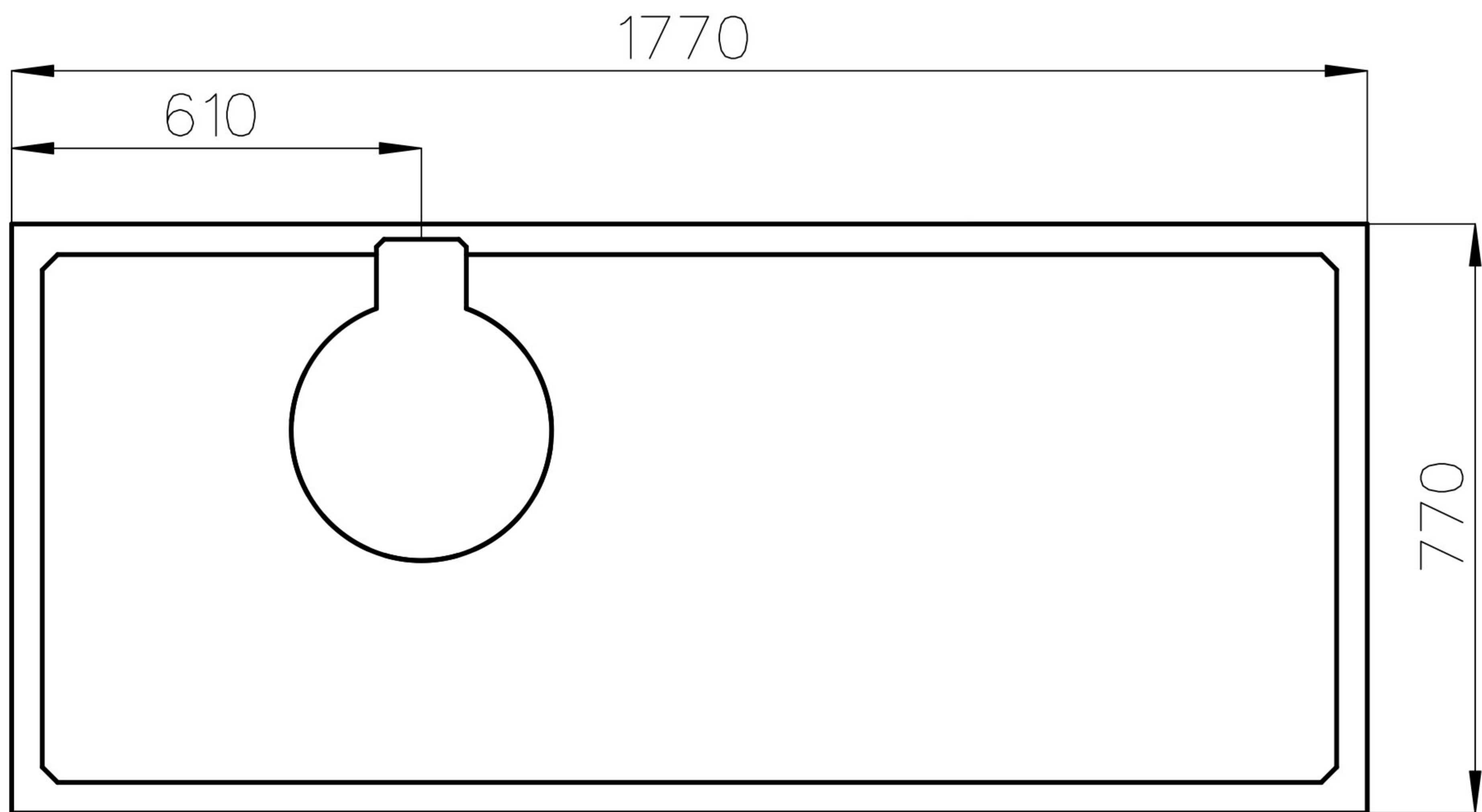
Draufsicht
