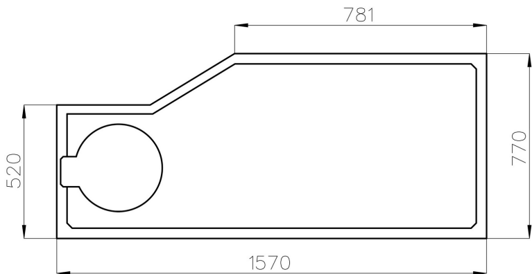
Draufsicht
