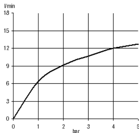
Durchflussdiagramm
