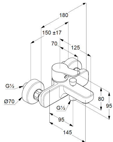
Maßzeichnung
