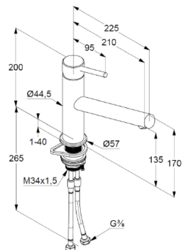
Maßzeichnung
