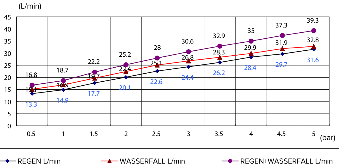
Abbildung - Durchflussdiagramm für die Regenpaneele 3870 und 3873.
