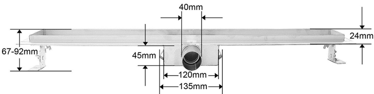
Typ - K: Bodenbefestigung mit umlaufenden Fliesenflansch
