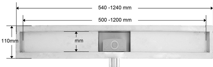
Typ - K: Bodenbefestigung mit umlaufenden Fliesenflansch
