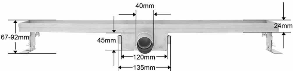
Typ - M: Bodenbefestigung ohne Fliesenflansch
