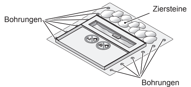
Abbildung E Anordnung der Ziersteine
