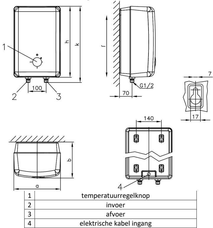
Afmetingen installatie (mm)
