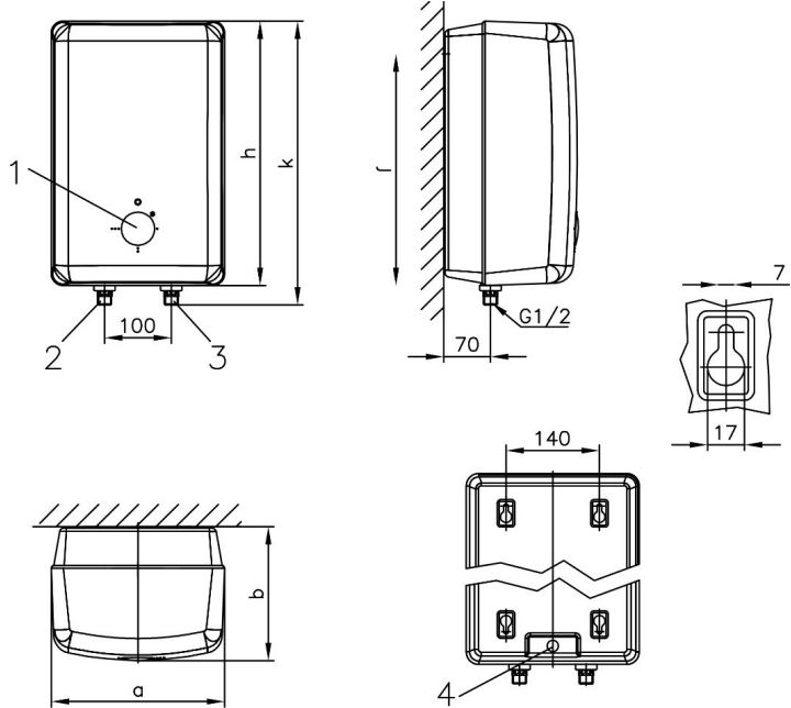
Wymiary montażowe (mm)
