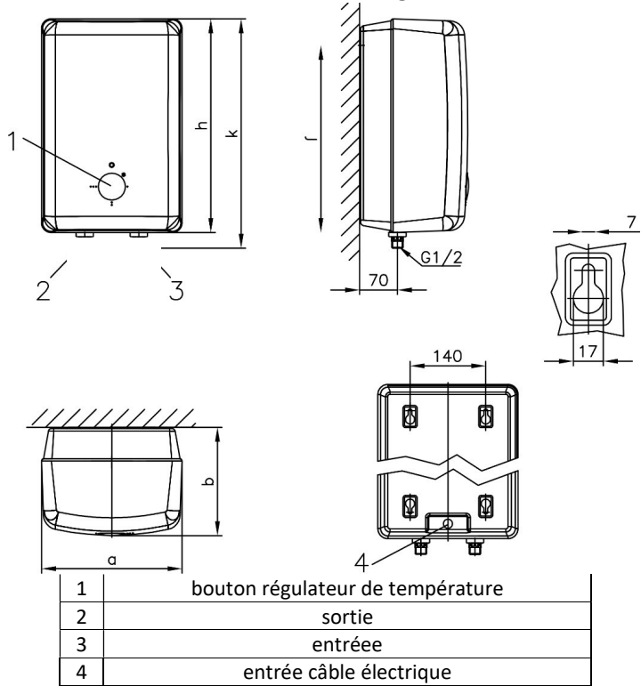
Dimensions de montage (mm)
