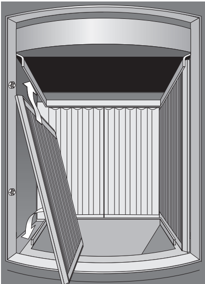
4. Feuerraumseitenwand einsetzen
