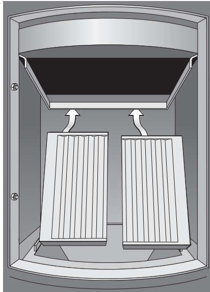
2. Feuerraumrückwände einsetzen
