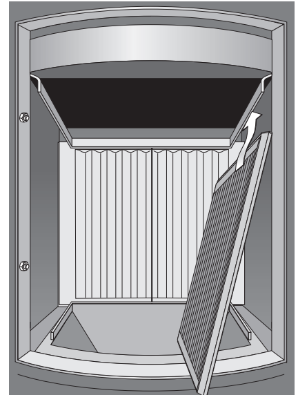
3. Feuerraumseitenwand einsetzen
