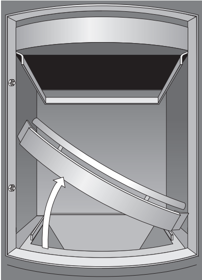
1. Stehrost entfernen
