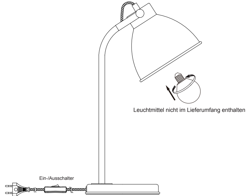
Montagezeichnung
