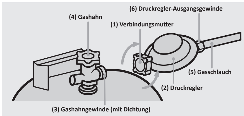
Abb.1: Montage des Druckreglers
