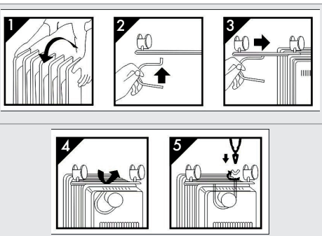
Abb.1: Montage Räder
