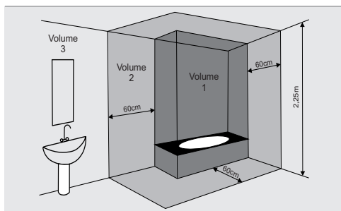
Abb.1: Sicherheitsabstände
