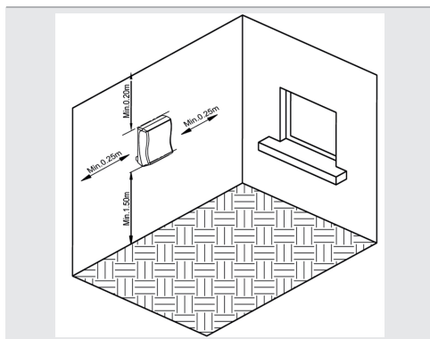
Abb.2: Montagemaße
