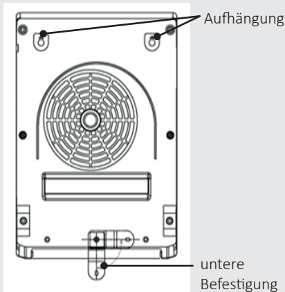
Abb.4: Anbringung
