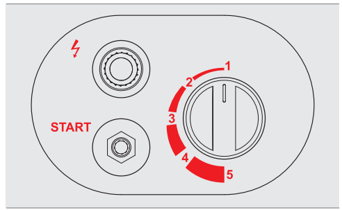
Abb. 5b: Bedienfeld (mit Thermostat)
